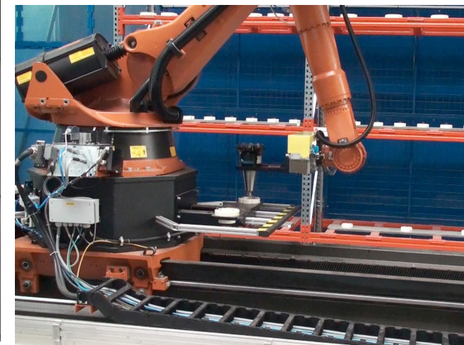
Ukládání nástroje do přechodného zásobníku na robotu
