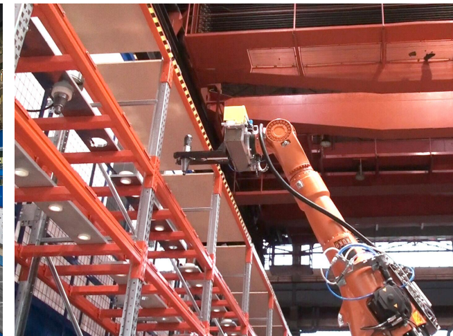
Vyjímání nástroje z regálového skladu
