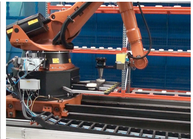
Werkzeugspeichern in der vorübergehenden Verwahrung an Roboter
