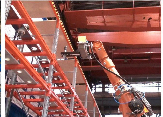
Toolsabnehmen aus dem Hochregallager
